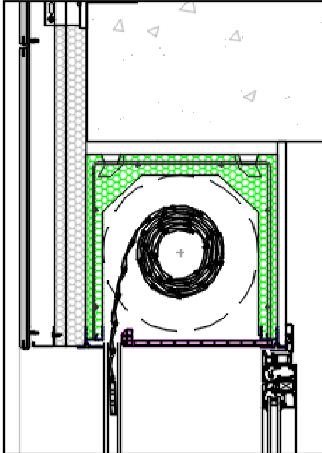
Fachada ventilada
