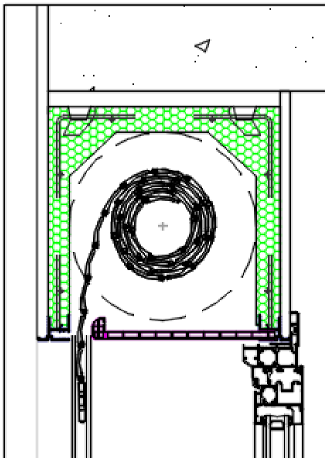
Revoco tradicional
