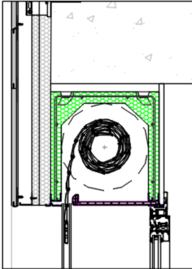
Fachada ventilada
