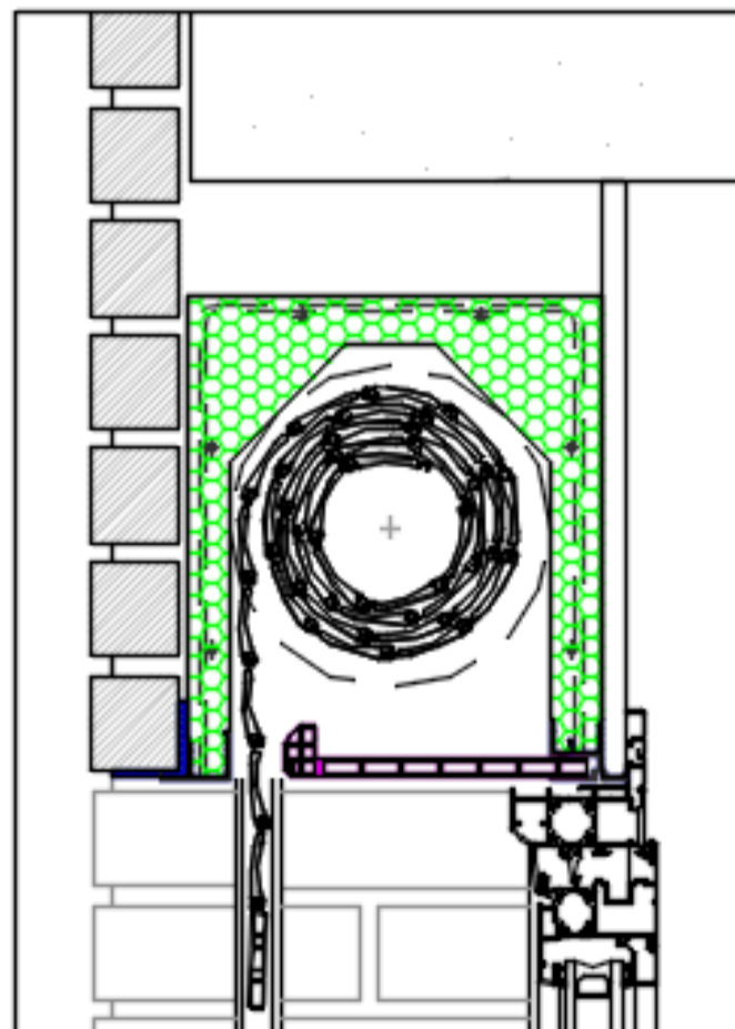
Obra vista
