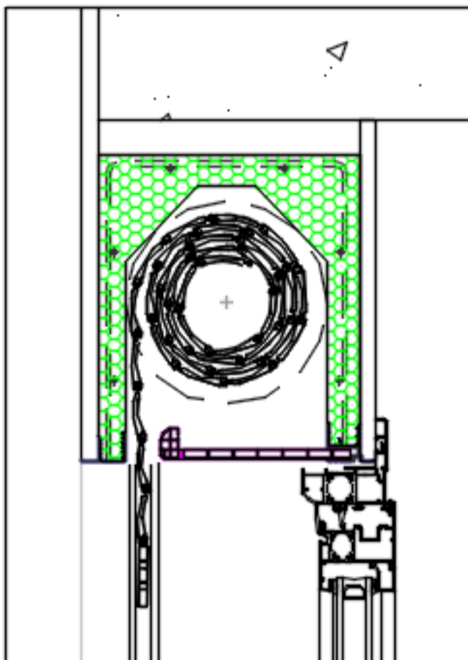
Revoco tradicional
